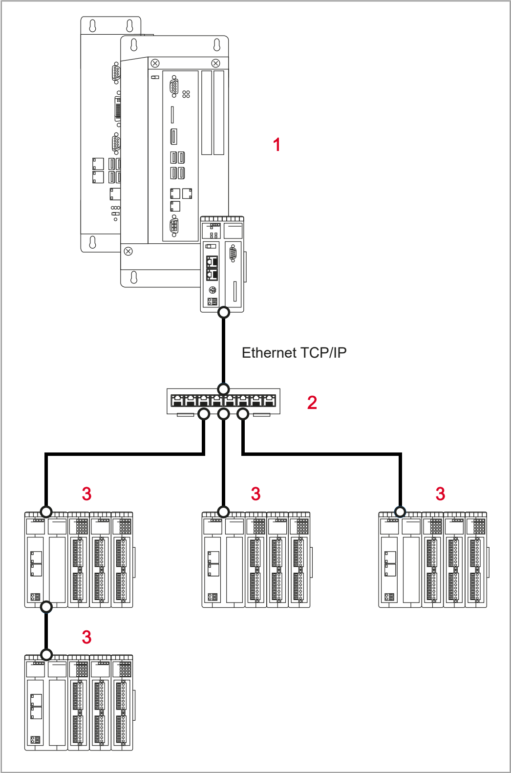
Abb. 14: Systemübersicht
