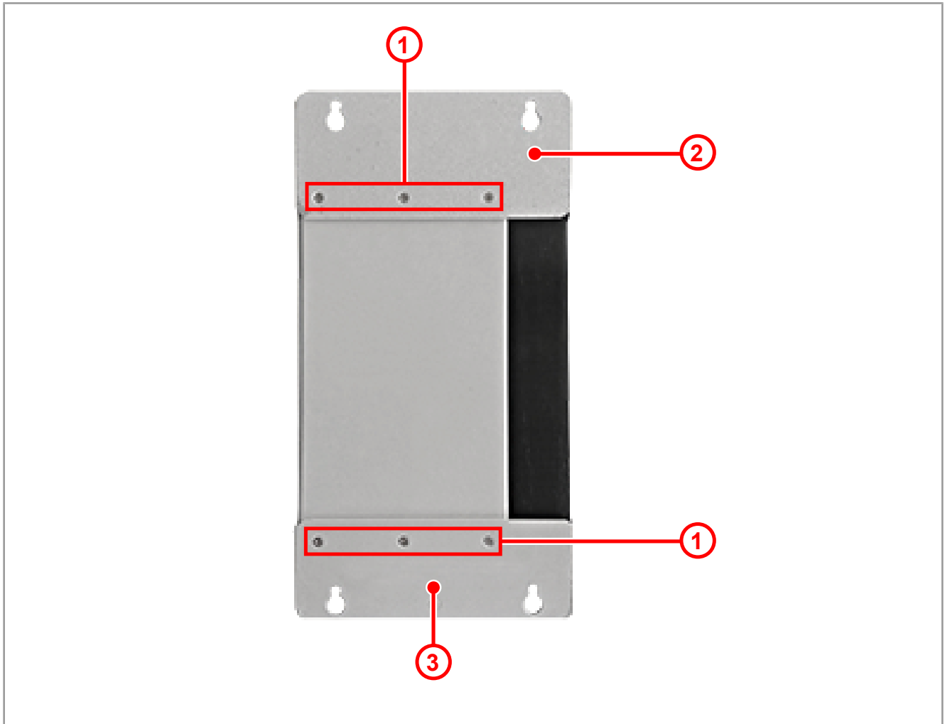
Abb. 7: JC-96x mit Originalbefestigungslaschen
