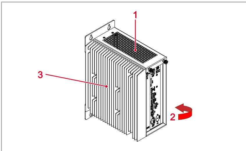
Abb. 2: Aufbau Gehäuse
