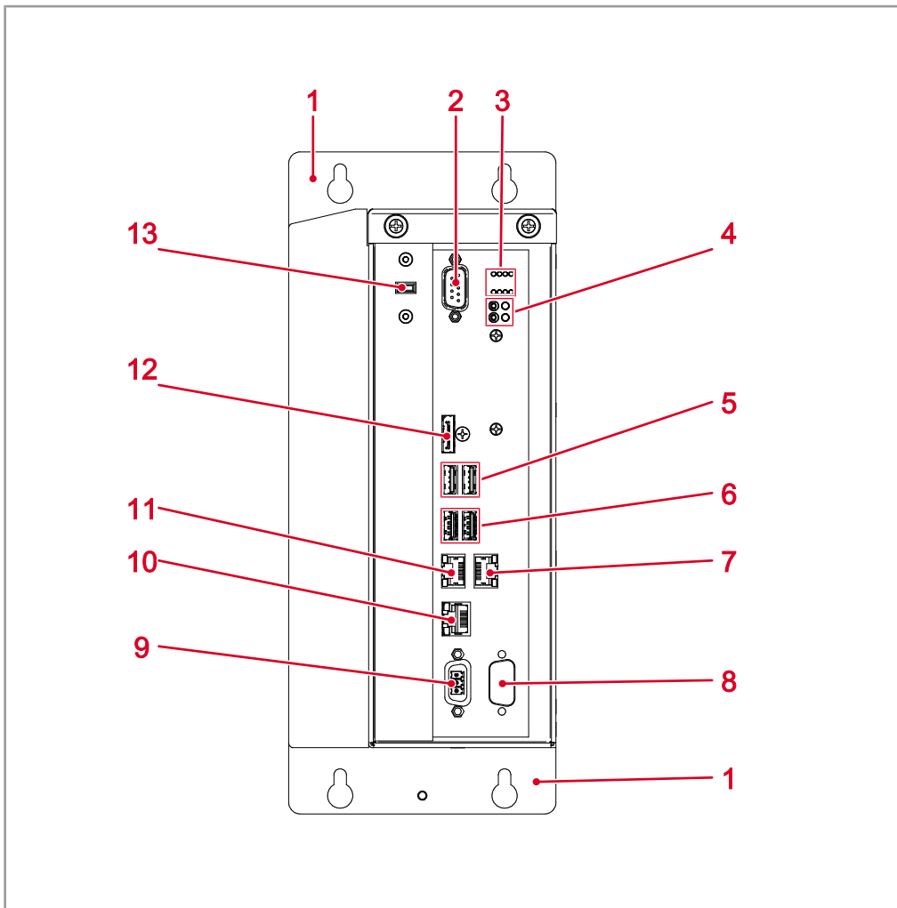
Abb. 1: Aufbau Front
