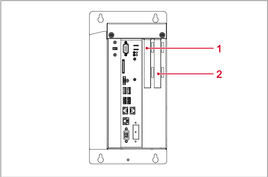
Abb. 7: PCI-Express-Bussteckplätze
