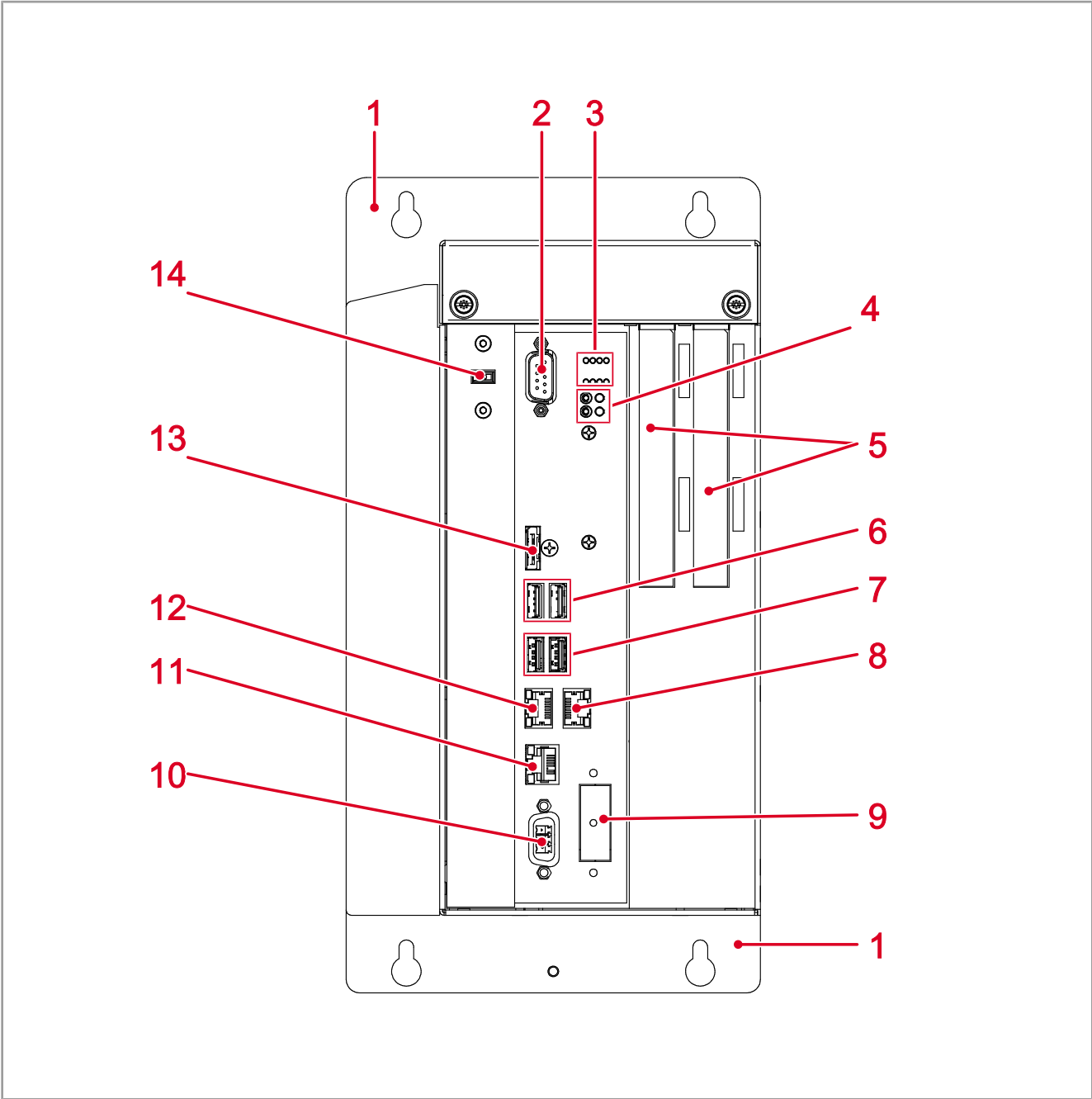
Abb. 1: Aufbau Front
