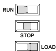
Abb. 13: Schalterstellungen S11
